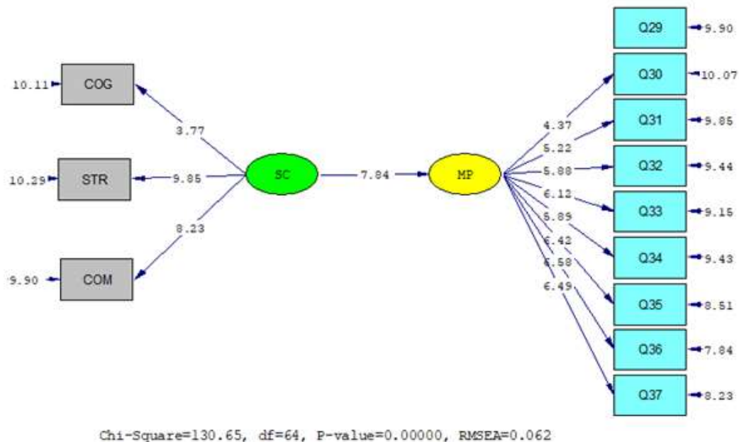
نمودار ۳. مدل ساختاری تحقیق فرضیه اصلی در حالت معناداری
