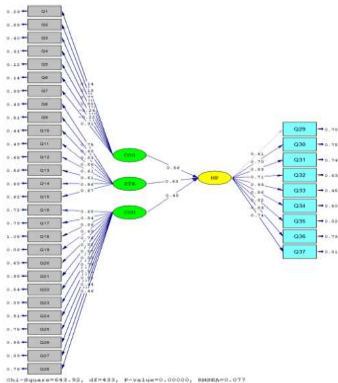
نمودار 5. مدل ساختاری تحقیق فرضیات فرعی در حالت استاندارد
